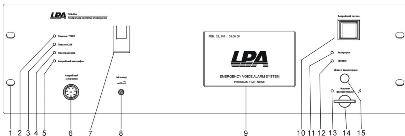
Рис. 3.2. Лицевая панель контроллера LPA-EVA-MA
