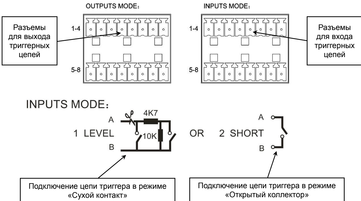
Рис. 4.44. Внешний вид разъемов и схема подключения цепей триггерных сигналов, расположенные на задней панели устройств LPA-EVA
